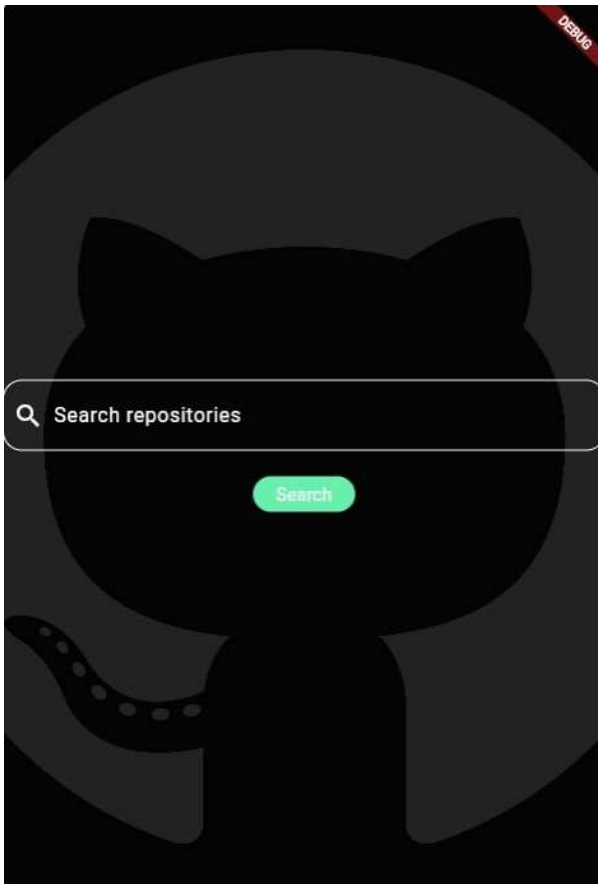
Slika 17 Početni zaslon
