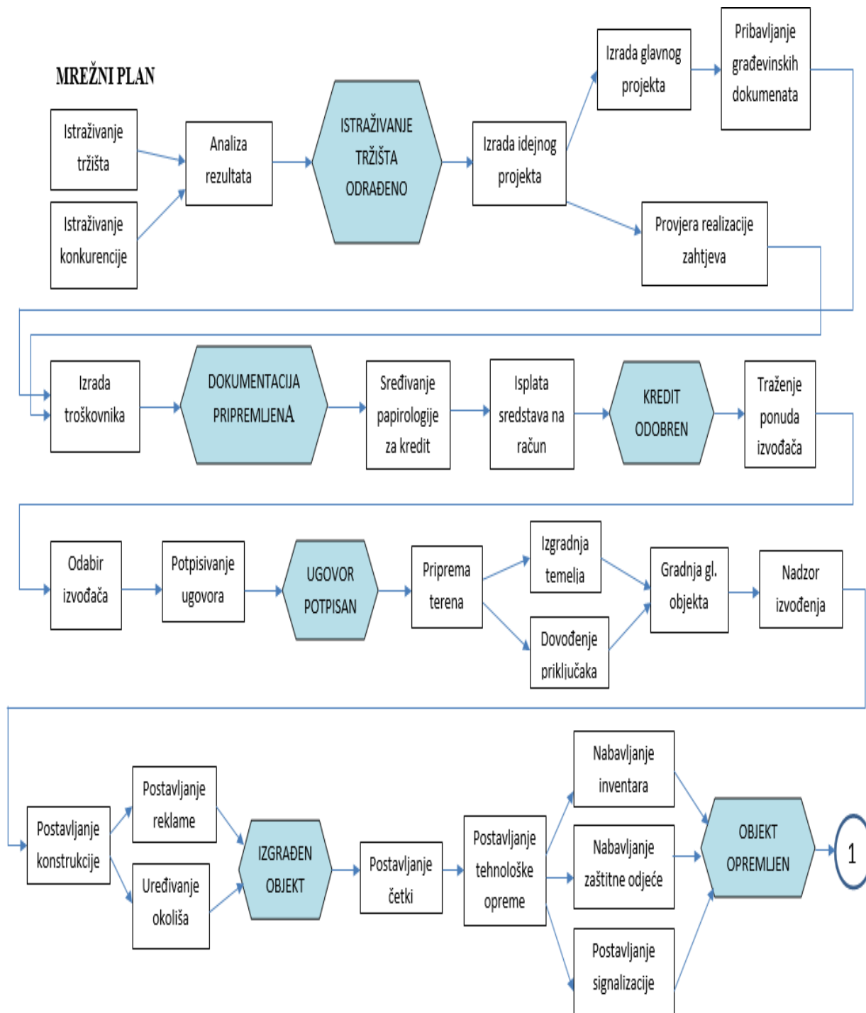
Slika 12 Mrežni plan 1/2
